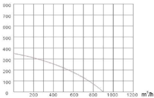
CDR2E-160
