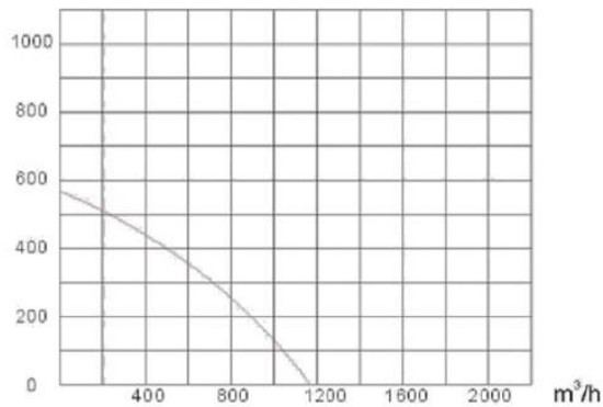
CDR2E-250
